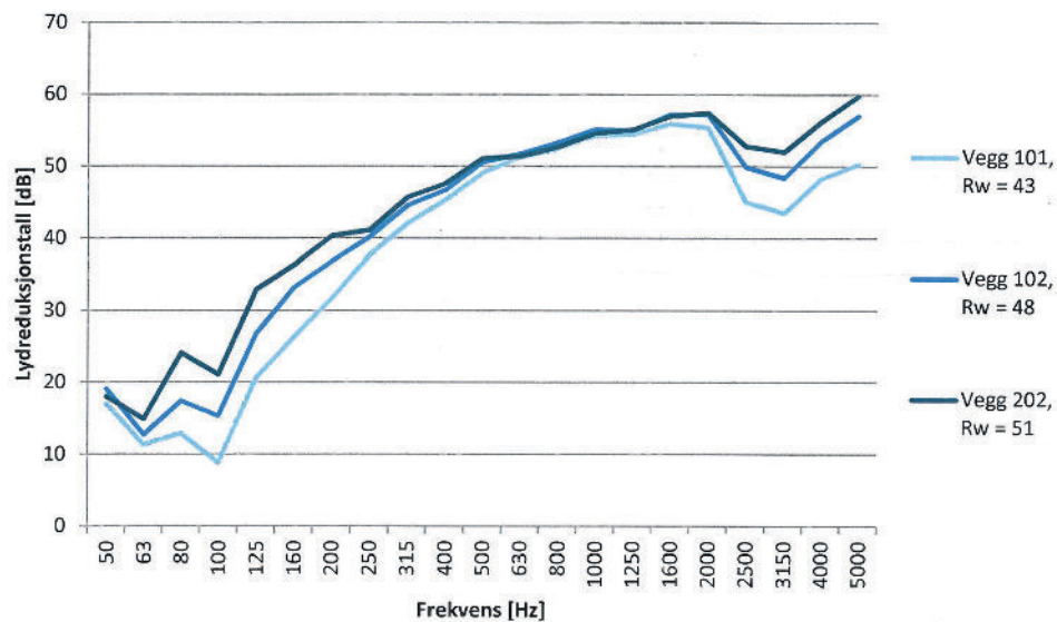
Diagram 1: Grafisk fremstilling av måleresultater i tredjedelsoktavgbånd for de tre veggene
